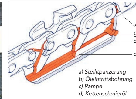
Patentiertes STIHL - Kettenschmiersystem für lange Lebensdauer
