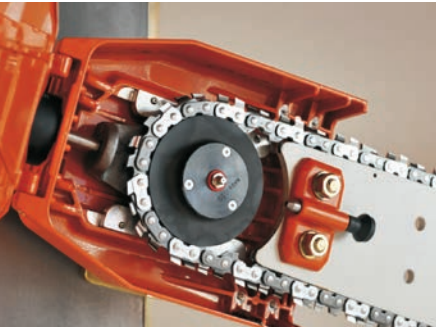
Changement rapide de la chaîne, sans outillage spécial
