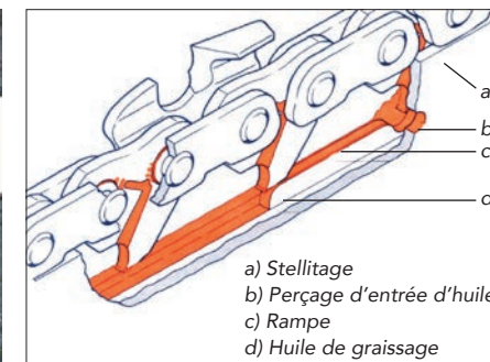
Système de graissage de chaîne STIHL-breveté pour une longue durée de vie
